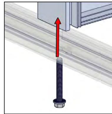
MFY-BOLT-3/8-16-2.5
